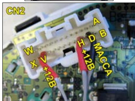
Питание D: масса; H,V: +12В
