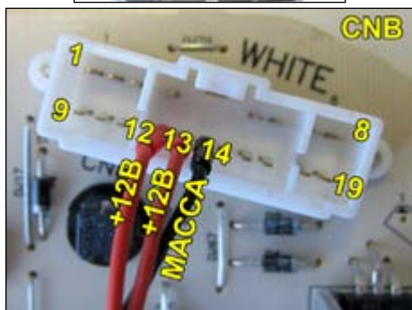
Питание 14: масса; 12 и 13: +12В
