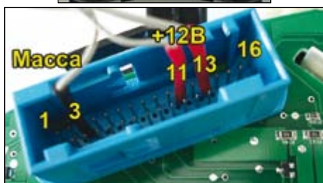
Питание 3: масса; 11 и 13: +12В
