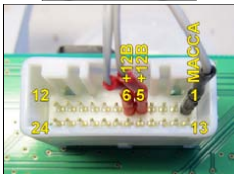
Питание 1: масса; 5, 6: +12В
