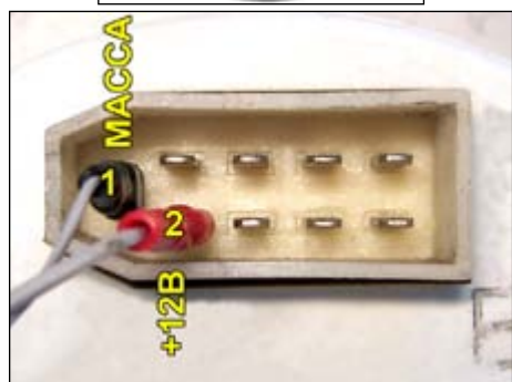
Питание 1: масса; 2: +12В
