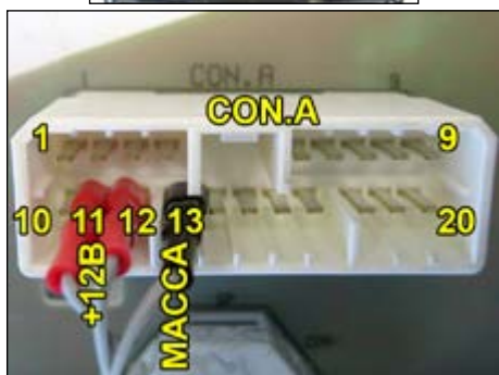
Питание 13: масса; 11 и 12: +12В
