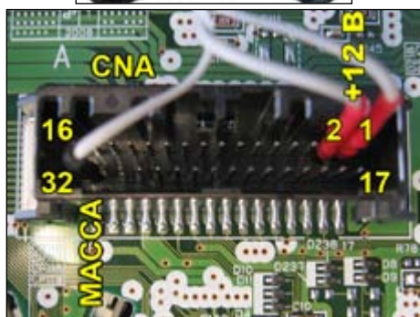
Питание 32: масса; 1 и 2: +12В
