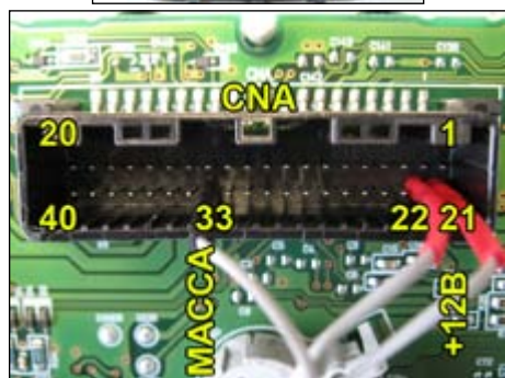
Питание 33: масса; 21 и 22: +12В
