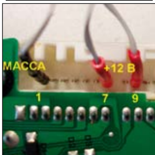
Питание 1: масса; 7 и 9: +12В
