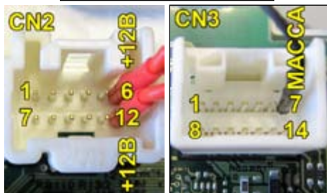
Питание CN3 - 7: масса; CN2 - 6 и 12: +12В
