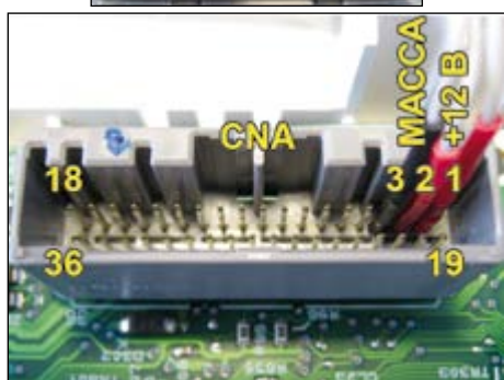
Питание 3: масса; 1 и 2: +12В
