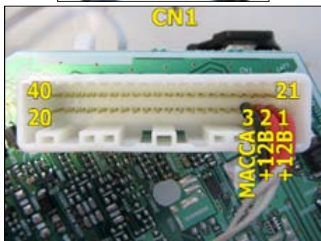
Питание 3: масса; 1, 2: +12В
