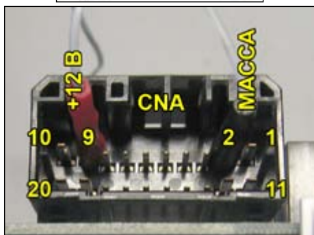
Питание 2: масса; 9: +12В
