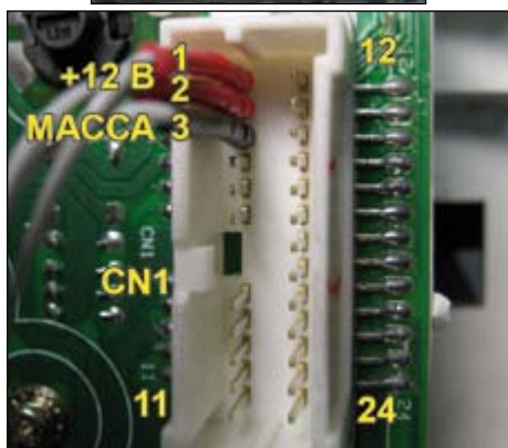
Питание 3: масса; 1 и 2: +12В
