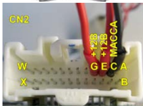
Питание E: масса; G: +12В
