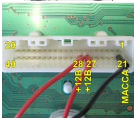
Питание 21: масса; 27, 28: +12В
