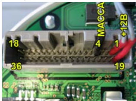
Питание 4: масса; 1 и 19: +12В
